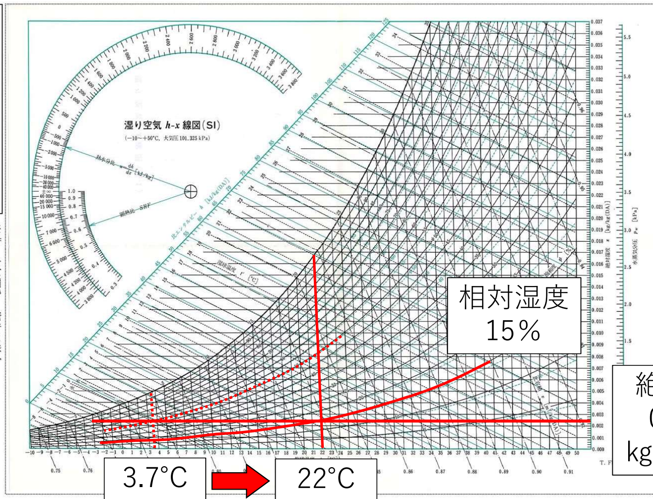
付図一 1 湿り空気線図 (h-x 線図)
